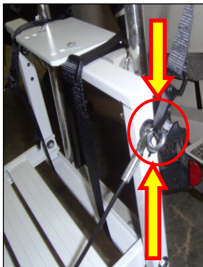
FIG. 4B EYE BOLT
